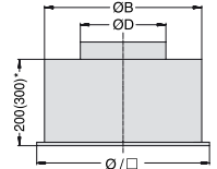
VDW-Q/R-...-V
