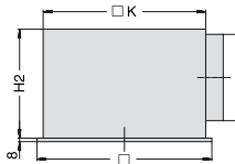
VDW-Q-...-H
