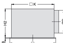
TDF-SA-Q-...-H
